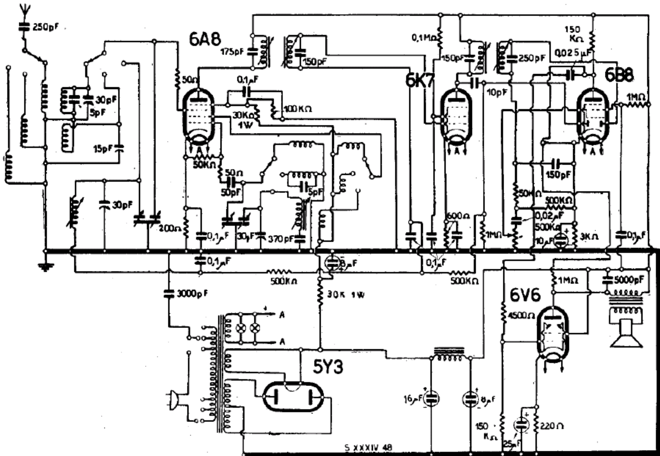
RADIO SUPERLA - MODD. « 532 » « 1532 FONO »
